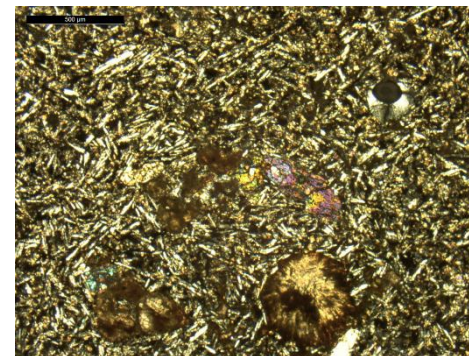
Étude pétrographique d'un boulet de calibre 116 mm en basalte, épave Mortella III .
